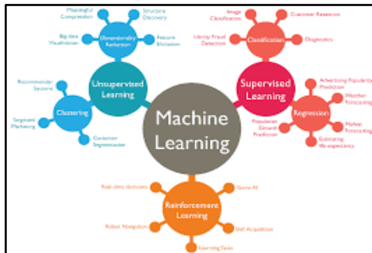
Gambar 4.4: Machine Learning(MalickSarr, 2021)
