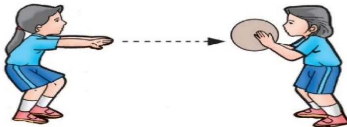
Gambar 5.11 Gerak Manipulatif
