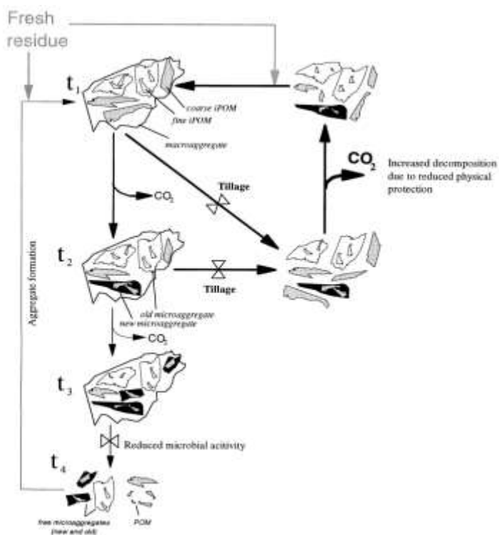
Gambar 2.1 Model konseptual yang menunjukkan cycle life macroaggregate dan pembentukan microaggregates. IPOM = partikulat bahan organik intraaggregate; POM = partikulat bahan organik; T waktu; \text{---}\text{X}\text{---} = Tingkat proses modifikasi (Six et al. , 2000)
